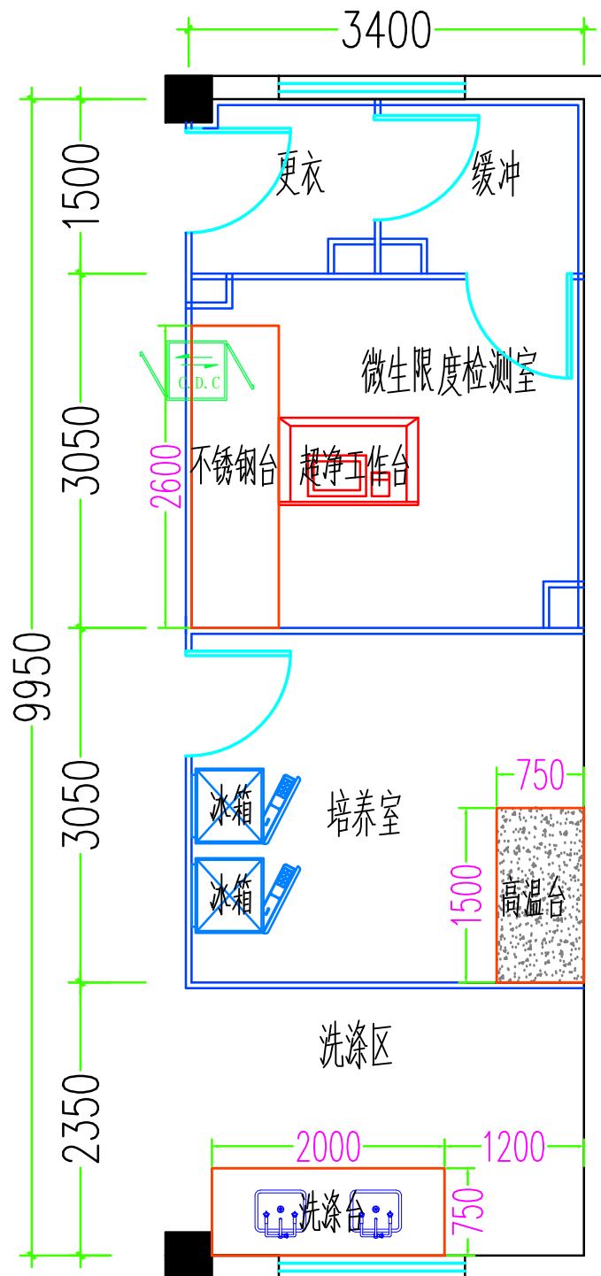
微生物实验室平面布局图
