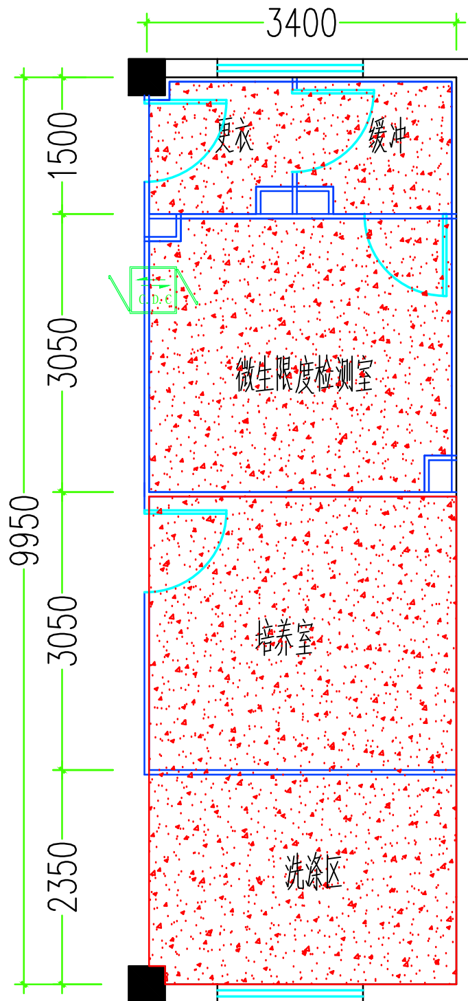
微生物实验室PVC地板胶平面图
