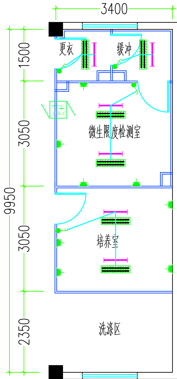
微生物实验室电气照明平面图
